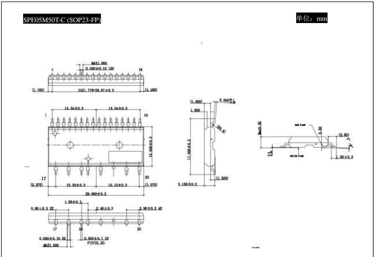
图 11: SPE05M50T-C 封装外形图
